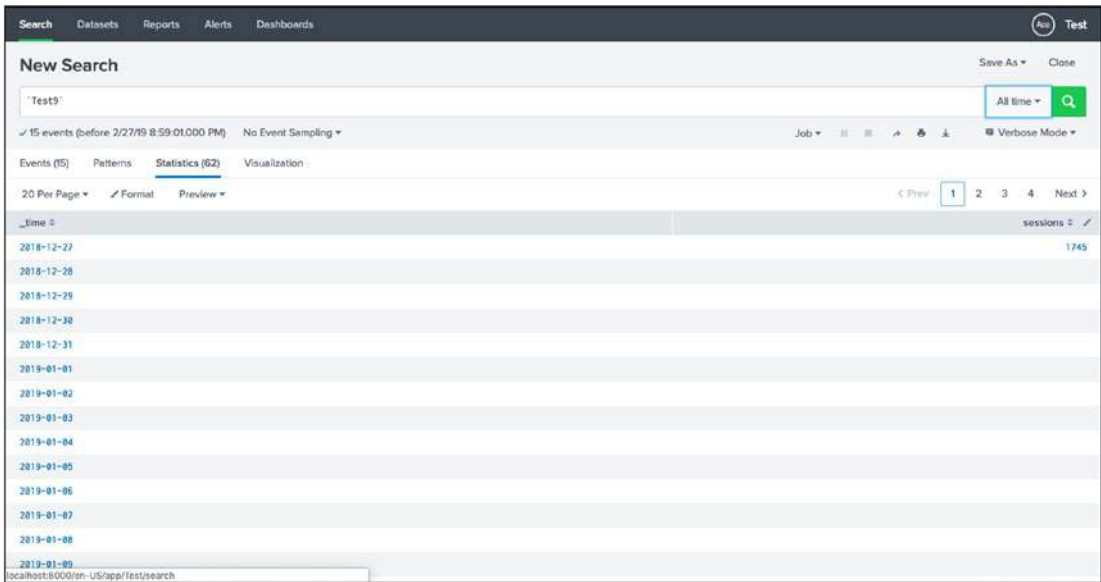
Figure 3-9. macro Test9
